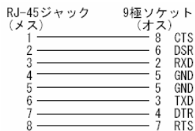
RJ-45 8 極ジャック ピン配置 (プラグ挿入方向より見る)
